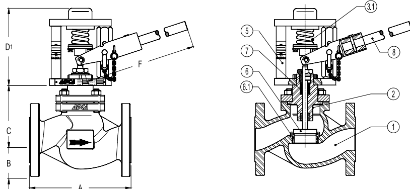
VPA26S– только ручное управление
