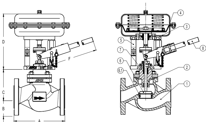
VPA26S– с пневматическим приводом и ручным управлением
