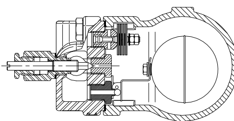
FLT17LC-FLT41 DN15-20
